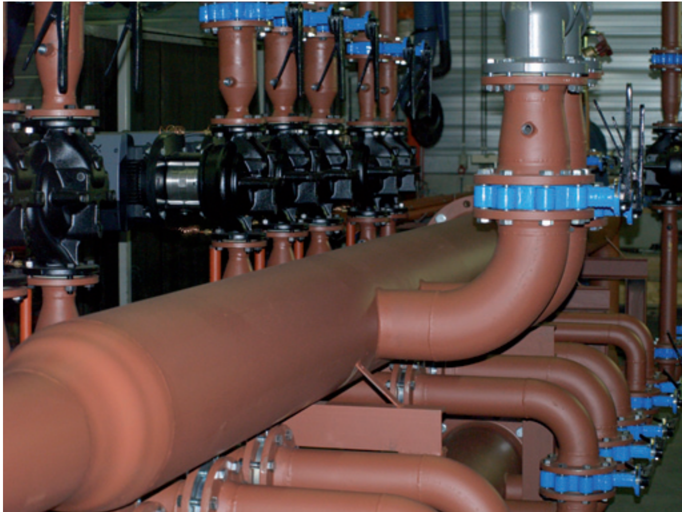
Montagewerkzaamheden: luchtkanalen Travaux de montage de Canalisations d'air
